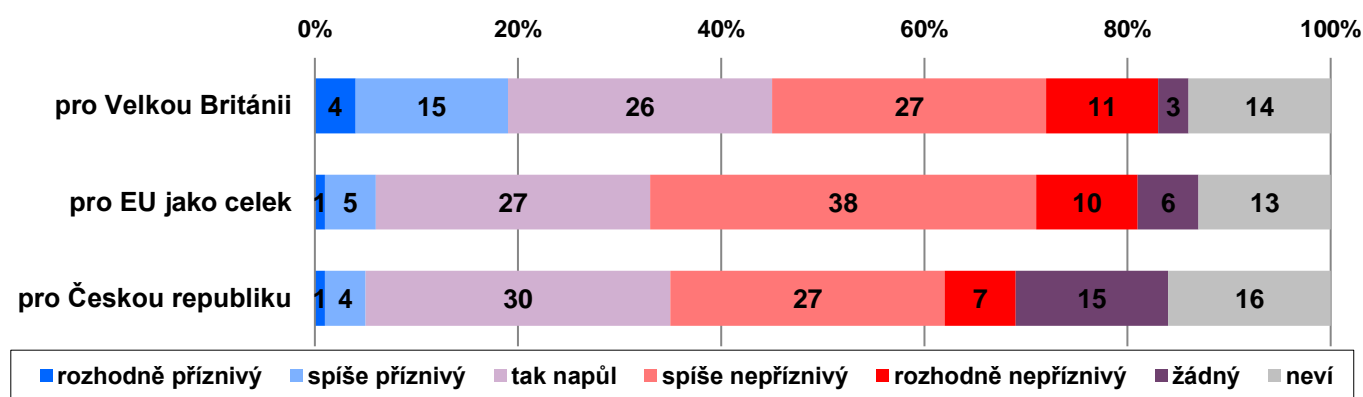
Graf 4: Dopady odchodu Velké Británie z EU 4
