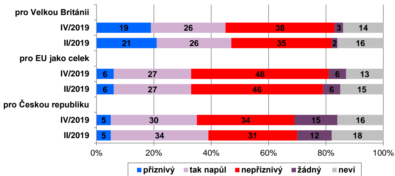
Graf 5: Dopady odchodu Velké Británie z EU – časové srovnání (v %)
