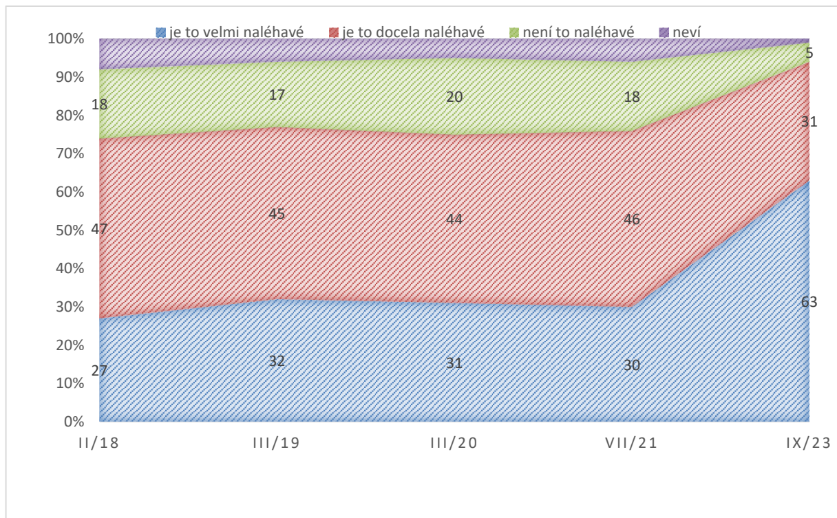
Graf 3ad: Naléhavost zabývat se zdroji, výrobou a distribucí energie – časové srovnání (%)
